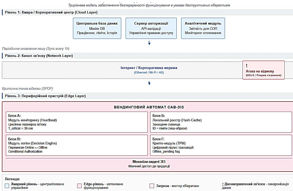
Рис. 2. Архітектурна схема гібридної кіберстійкої системи CAB-313
