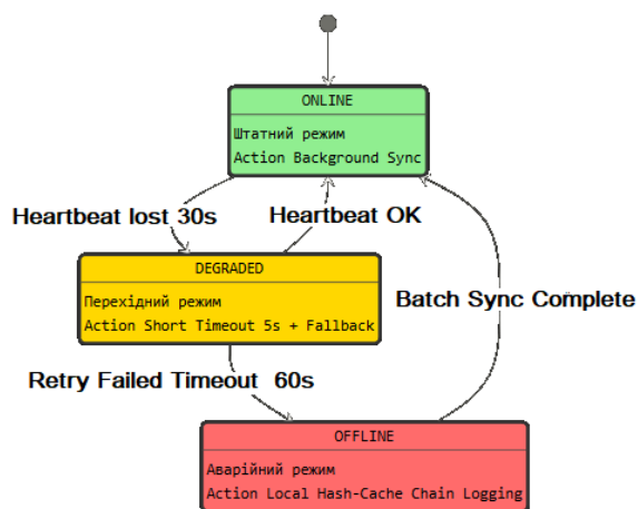
Рис. 1. Діаграма станів (Finite State Machine) контролера CAB-313 та логіка переходів
